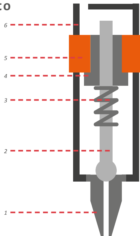
3A. Schema sezione interna dei componenti principali (a scopo puramente illustrativo)
